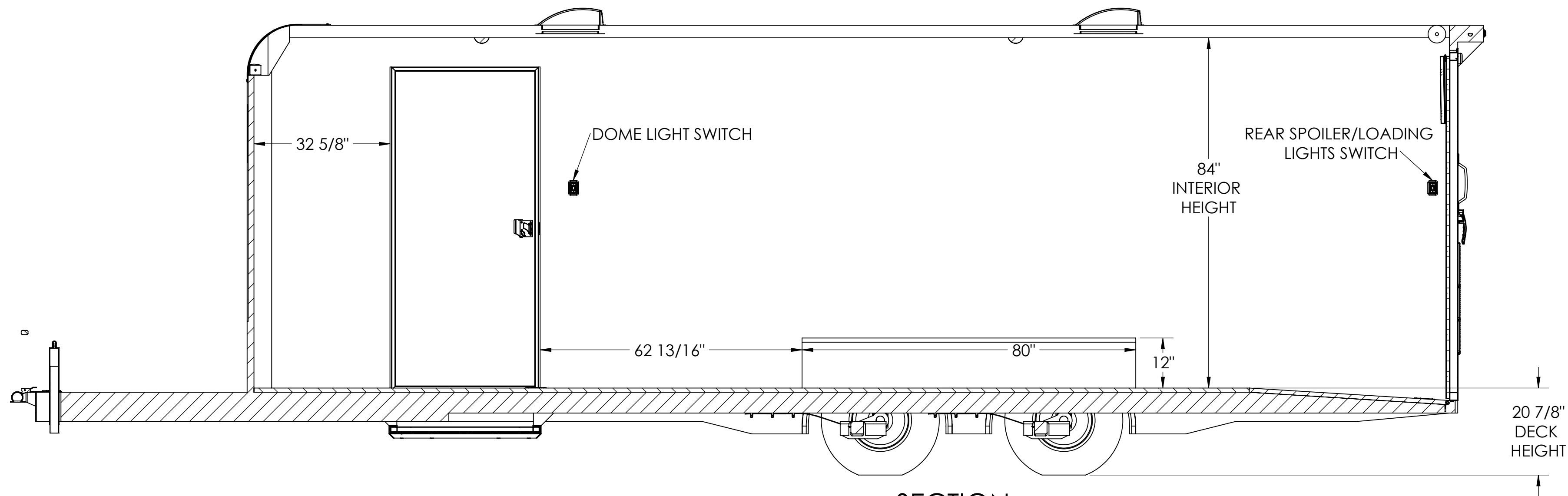
SECTION A-A SCALE 1 : 20
